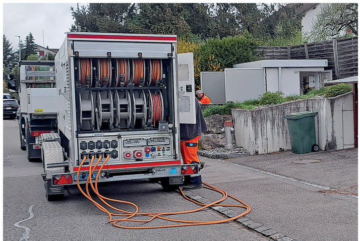
Einbau einer neuen Mittelspannungs- anlage in der TST Vorstadt in Laupersdorf
